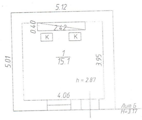
план 1 этажа
